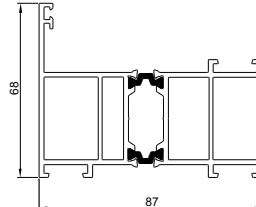
Profil prog ENERGY 90
