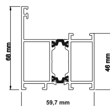
Profil prog ENERGY 60
