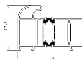
Profil ościeżnicy KMT ENERGY 90
