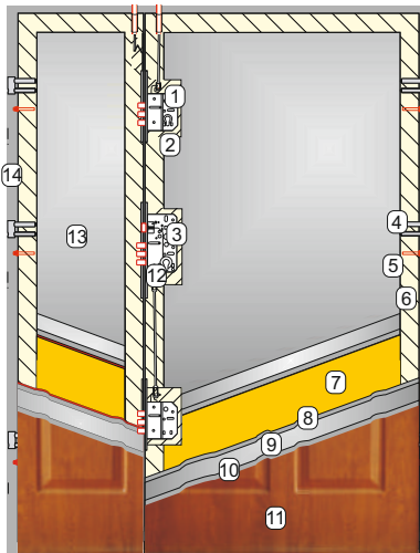
KMT PLUS 54 - dostawka otwierana
