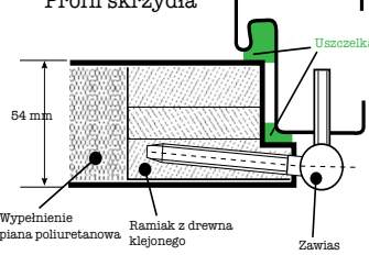
Profil skrzydła
