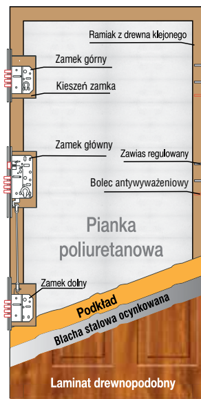
Profil skrzydła
