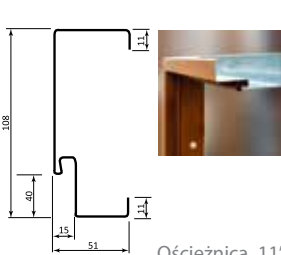
Ościeżnica „11”
