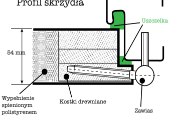
Profil skrzydła
