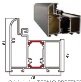
Ościeżnica TERMO PRESTIGE
