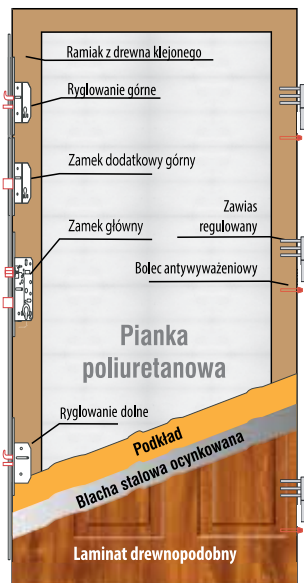
Profil skrzydła
