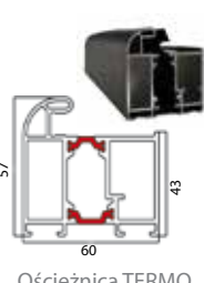
Ościeżnica TERMO
