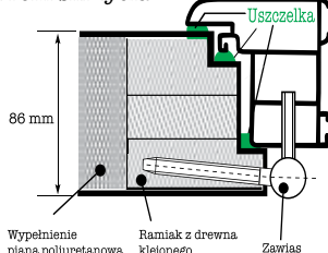
Profil skrzydła
