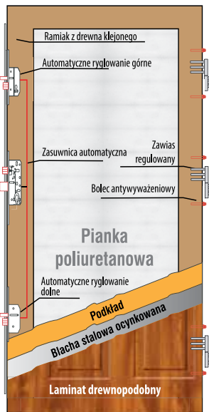
Profil skrzydła
