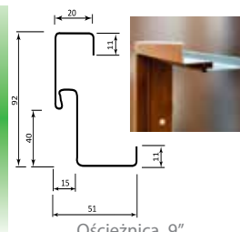
Ościeżnica „9”
