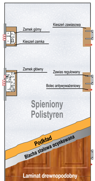
Profil skrzydła
